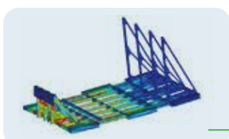
Analiza dynamiczna wózka do badań zderzeniowych
