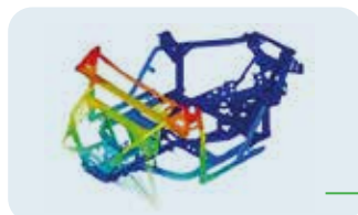
Analiza sztywności skrętnej ramy pojazdu
